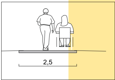
Prinzipschnitt Hauptweg, M 1 : 50
